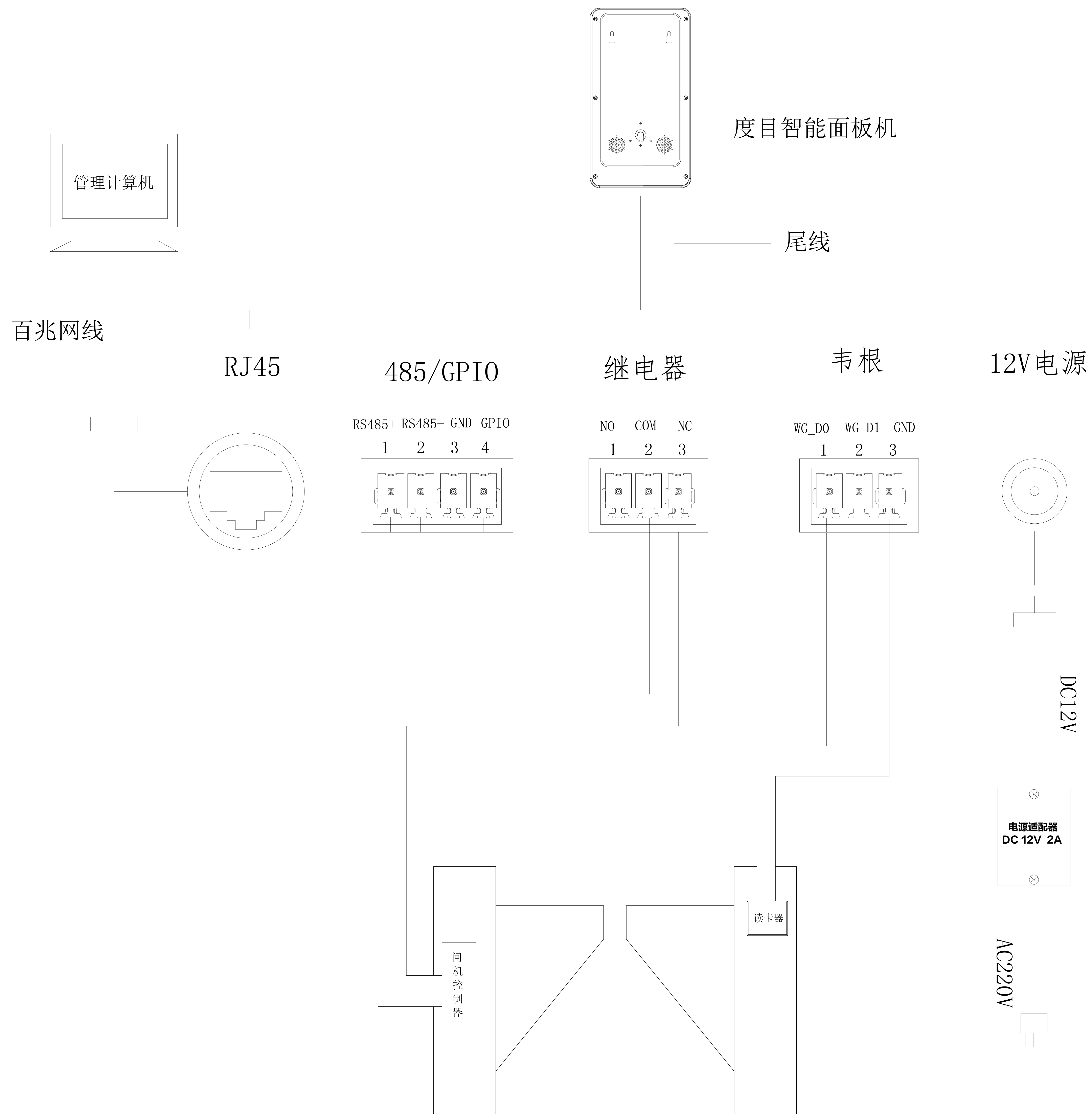
闸机门禁系统接线图
